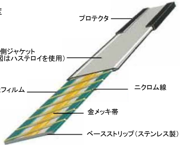
メトリテープ式液面計センサー イメージ図
